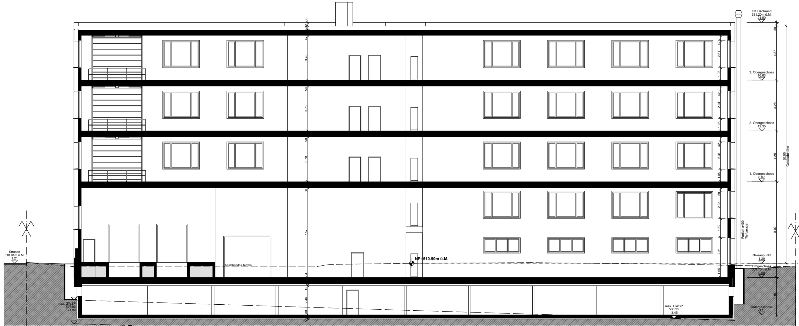
Schnitt E
