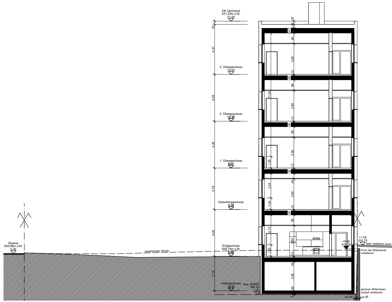
Schnitt F
